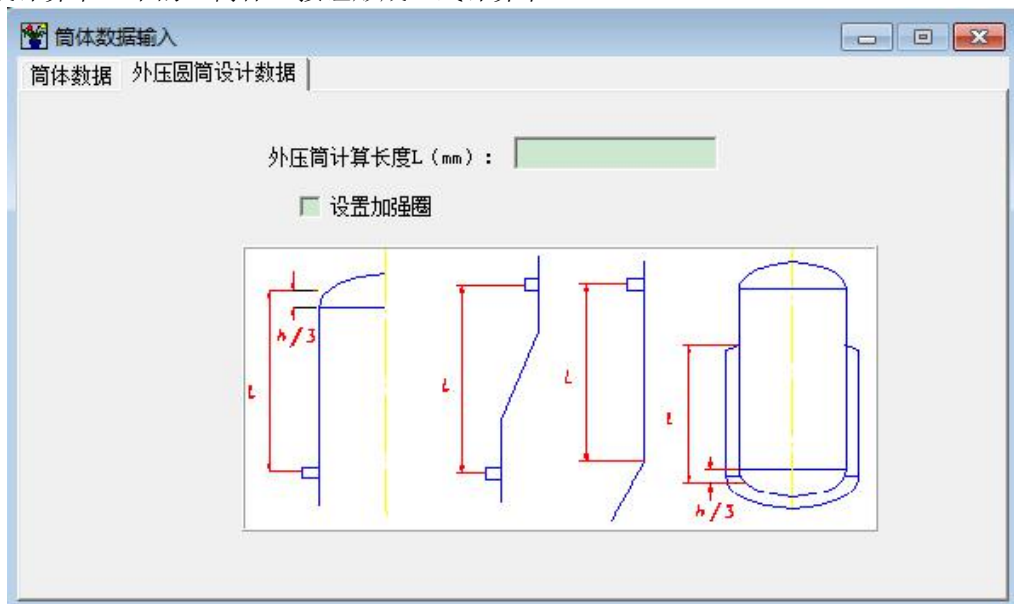
图 4.3 外压圆筒计算长度输入
