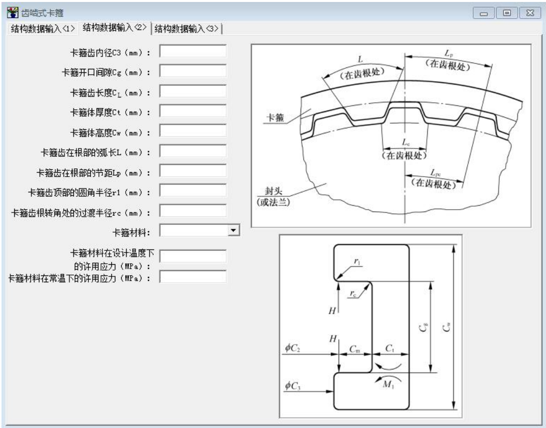
图 14.20 齿啮式卡箍结构数据输入（2）
