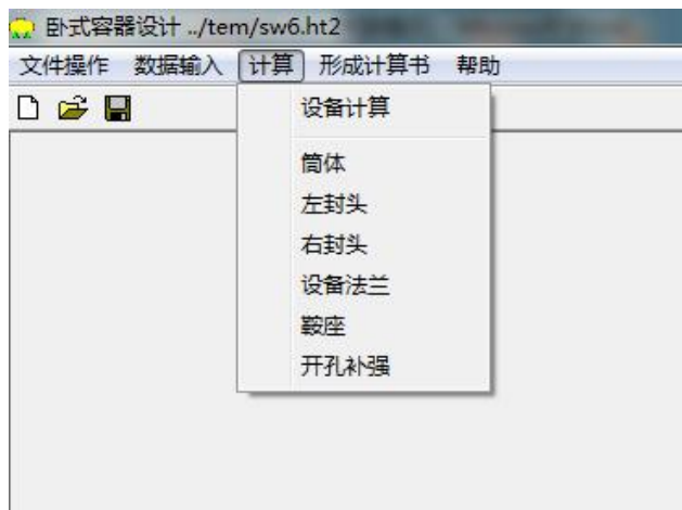
图 5.1 卧式容器数据输入和计算
