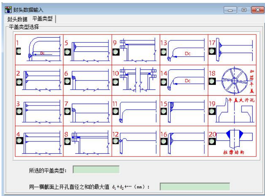
图 4.14 平盖结构类型选择
