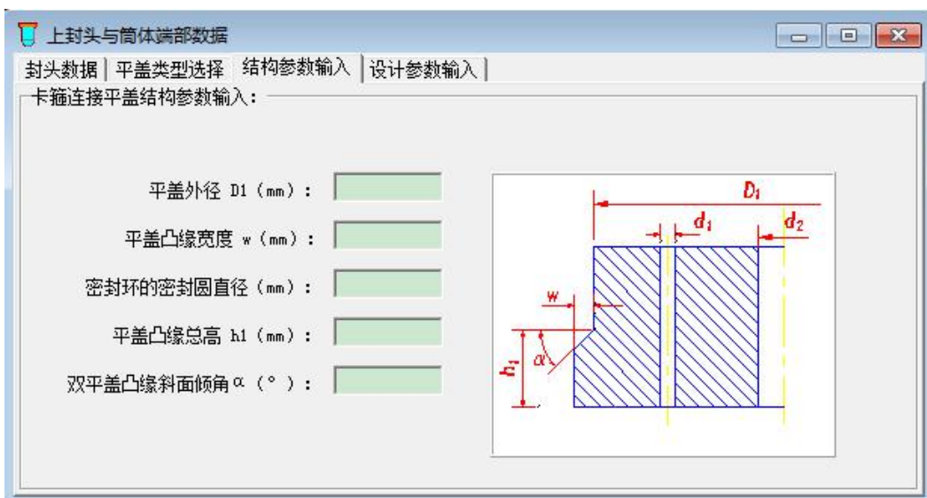
图 10.8 卡箍结构平盖数据输入
